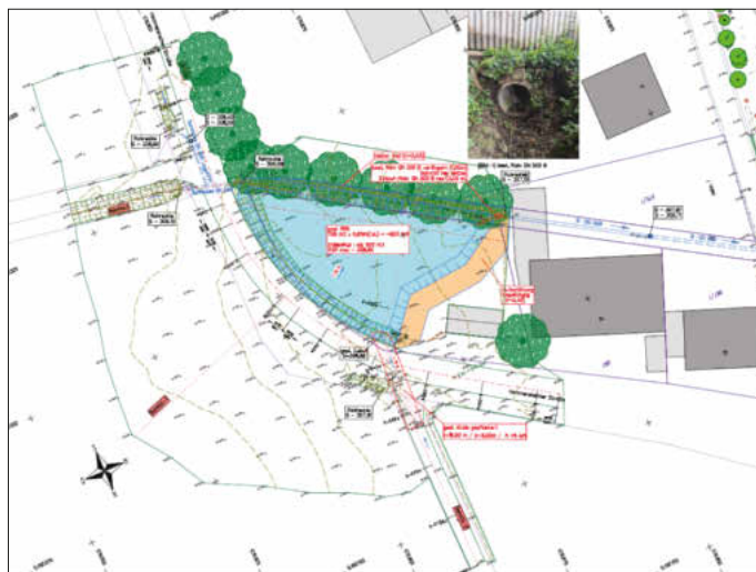
Erste Entwurfsplanung
